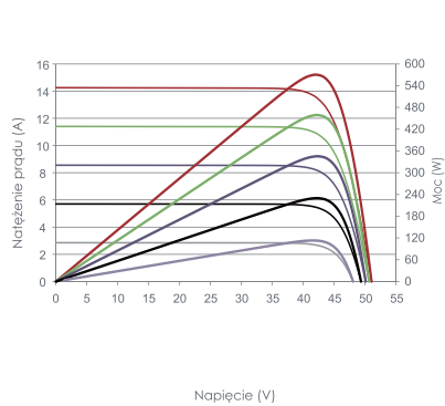
Krzywe charakterystyki prądowo-napięciowej i mocowo-napięciowej (590W)
