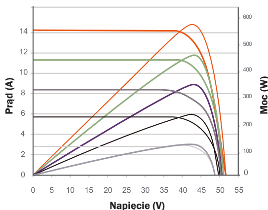
Charakterystyka elektryczna
